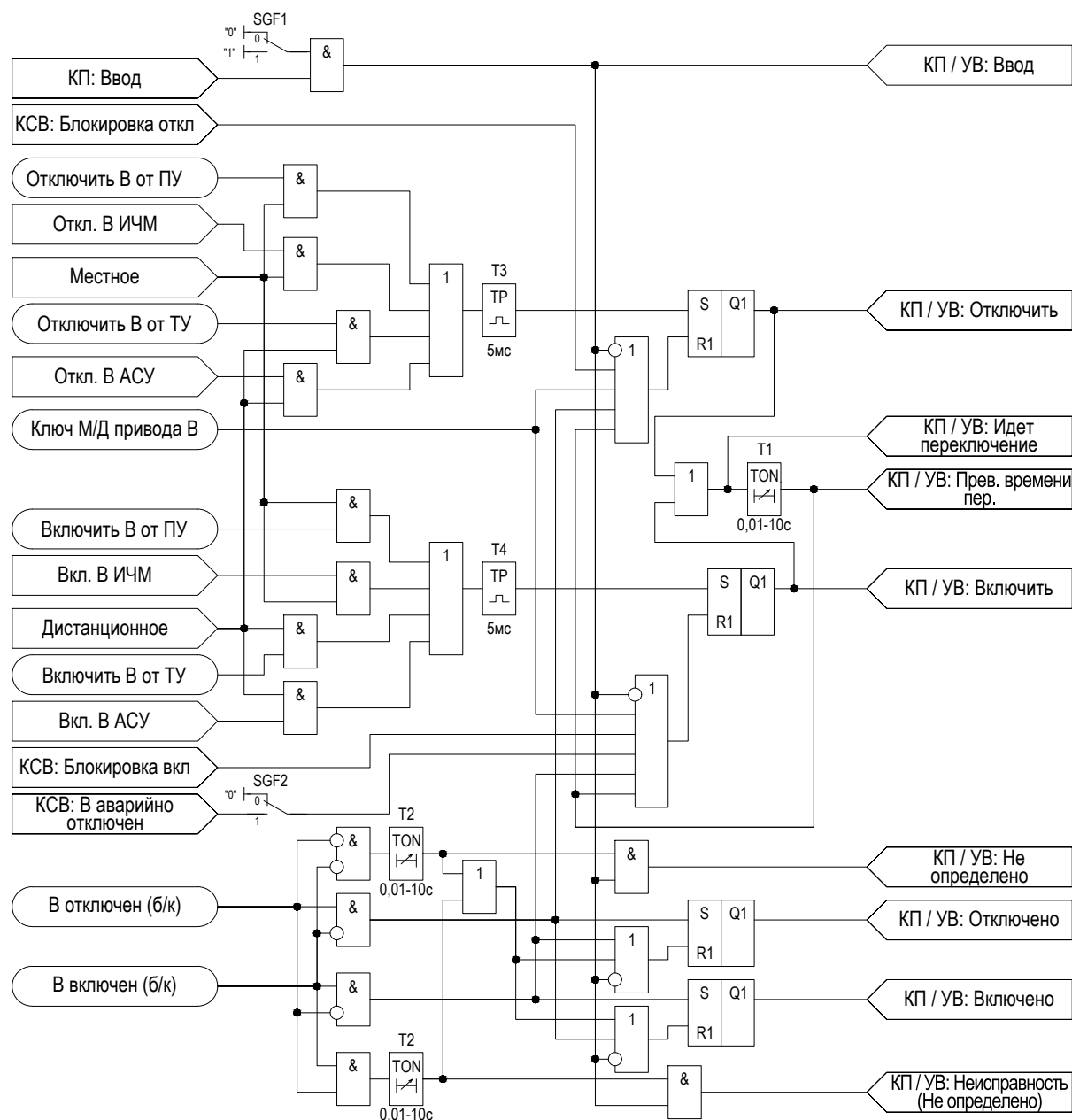
Рисунок 2.17 – Функциональная схема «УВ»
