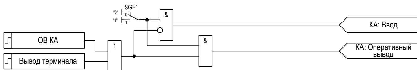
Рисунок 2.18 – Логика управления режимами функционального блока «КА»
