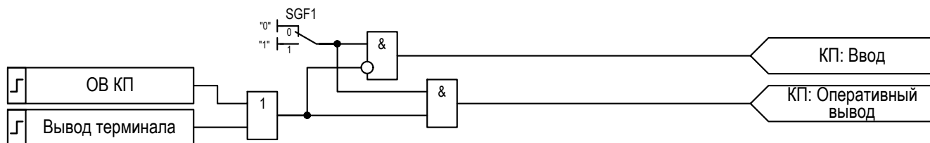
Рисунок 2.16 – Функциональная схема управления режимами работы «КП»
